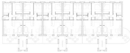
CONJUNTO VIVIENDAS EN TORRETA 1500 300PE LOCAL L-4-1 E. 1/100
