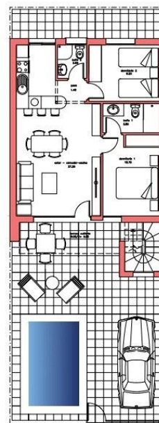
PLANTA BAJA
