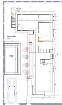
PLANTA BAJA
