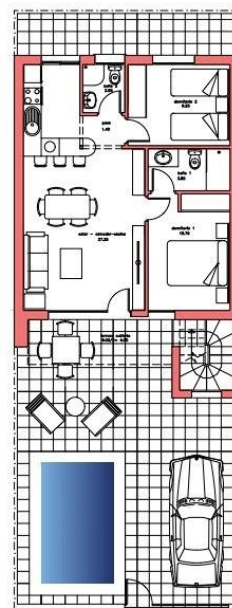
PLANTA BAJA
