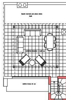
PLANTA SOLARUM
